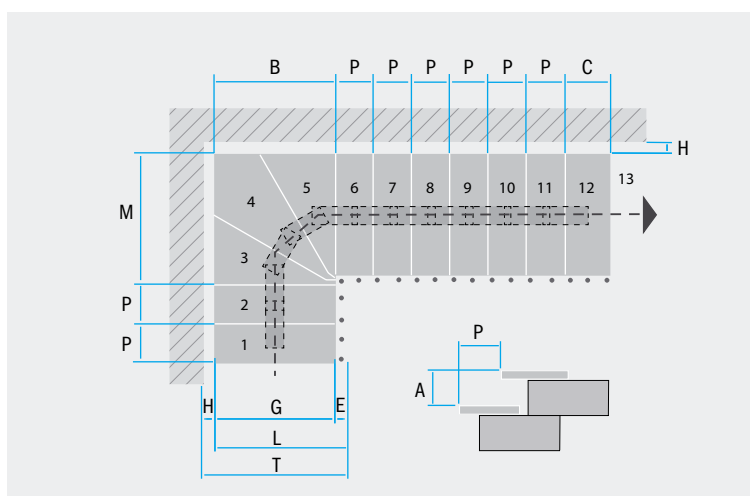
vista in pianta con ingombri
