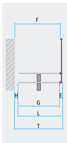
vista frontale con 1 lato di ringhiera
